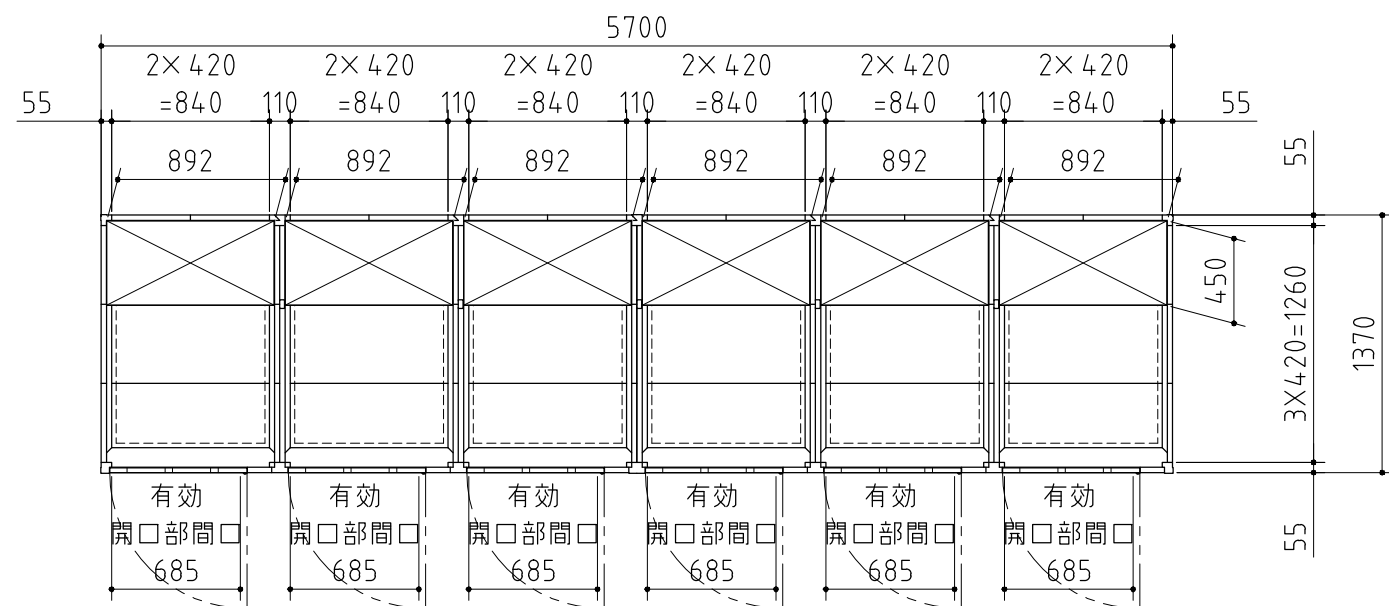
平面図
